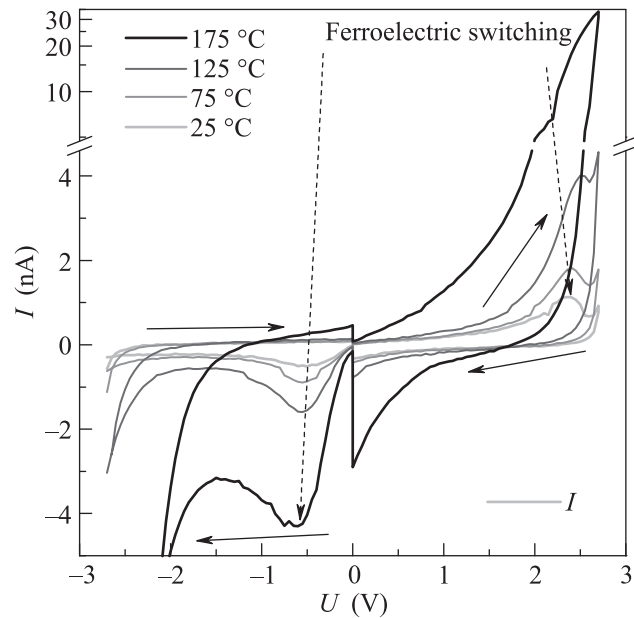
Рис. 3. Экспериментальные вольт-амперные характеристики структуры Pt/f-Hf 0.5 Zr 0.5 O 2 /TiN при различных температурах. Сплошные стрелки показывают направление развертки напряжения, штриховые – точки сегнетоэлектрических переходов
