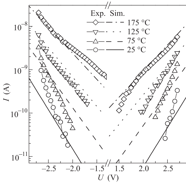
Рис. 2. Экспериментальные (символы) и рассчитанные (линии) вольт-амперные характеристики структуры Pt/a-Hf 0.5 Zr 0.5 O 2 /TiN при различных температурах
