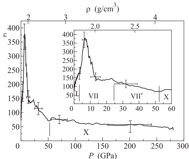
Рис. 3. Диэлектрическая проницаемость воды как функция давления при изэнтропическом сжатии с начальной температурой T = 280 К. На верхней оси показана плотность воды. На вставке – увеличенный фрагмент графика. Тонкими линиями условно показаны границы фаз; L – жидкая вода, римские цифры – фазы льда
