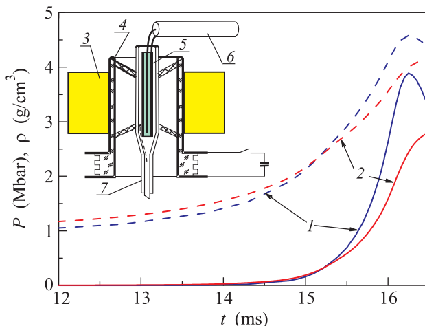
Рис. 1. (Цветной онлайн) Зависимость давления (сплошная линия) и плотности (штриховая линия) от времени в экспериментах со льдом (1) и водой (2). На вставке схематичное изображение установки: 3 – кольцевой заряд взрывчатого вещества, 4 – соленоид-оболочка, 5 – камера сжатия с образцом, 6 – коаксиальный кабель, 7 – криопровод для охлаждения образца
