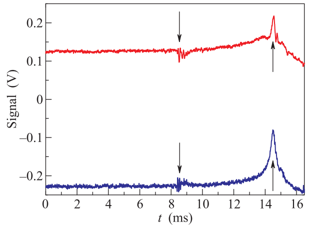
Рис. 2. (Цветной онлайн) Пара квадратурных сигналов рефлектометра в эксперименте с водой
