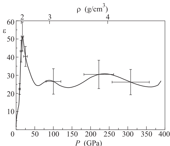
Рис. 4. Диэлектрическая проницаемость льда при изэнтропическом сжатии. Начальная температура T = 80 К
