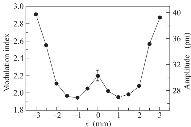
Рис. 2. Зависимость значения индекса модуляции m_c = 2\pi r_c / \lambda от положения отверстия свинцовой маски, которая перемещалась вдоль поверхности нержавеющей фольги. Значение x = 0 соответствует ее центру. На правой оси указаны соответствующие значения смещений в пикометрах
