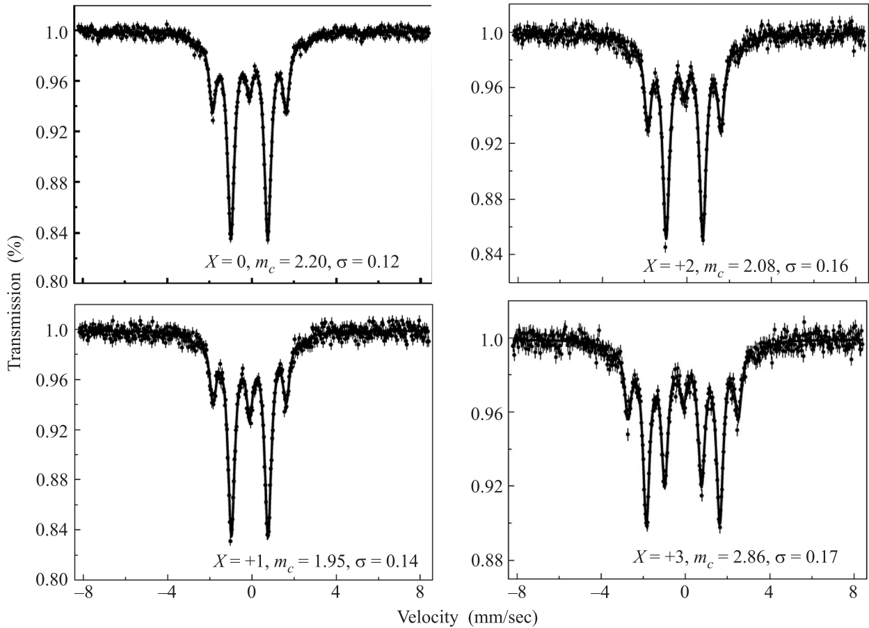
Рис. 3. Мессбауровские спектры фольги, полученные с использованием свинцовой маски с отверстием 0.6 мм. Положение отверстия x и значения параметров m_c и \sigma указаны на графиках. Точками показаны экспериментальные спектры, сплошными линиями – результаты теоретического моделирования
