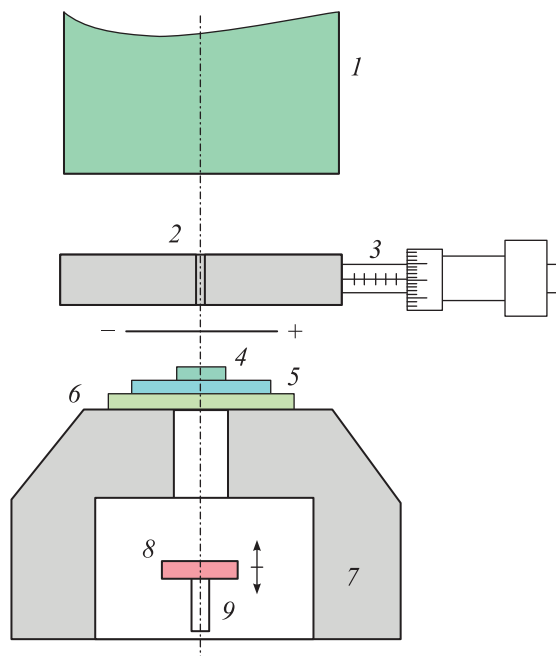
Рис. 1. (Цветной онлайн) Схема конструкции узла смещений. 1 – детектор; 2 – диафрагма в свинцовой пластине; 3 – микрометрический узел; 4 – образец; 5 – пьезопреобразователь; 6 – держатель из оргстекла; 7 – свинцовый коллиматор; 8 – мессбауэровский источник; 9 – шток мессбауэровского модулятора
