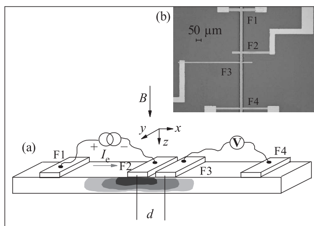
Рис. 1. (а) – Схема устройства для измерений электрических сигналов, обусловленных диффузией спин-поляризованных электронов. F1–F4 – ферромагнитные электроды, намагниченные вдоль оси y , расположенные на поверхности полупроводникового канала, в котором происходит спиновый транспорт. Ток I_e течет от F1 к F2, под электродом F2 условно затемнением с разной контрастностью показано облако поляризованных по спине электронов, степень поляризации которых по мере удаления от инжектирующего электрода убывает. Измерение нелокального напряжения производится между контактами F3 и F4. (б) – Фотография устройства с латеральными контактами. Вертикальная полоска – полупроводник InSb, наблюдаемый в окне размерами 50 \mu\text{м} \times 1.8 \text{мм} , сделанном в слое фоторезиста толщиной 1 \mu\text{м} . Канал из полупроводника пересекают четыре горизонтальных ферромагнитных контакта, отделенных от полупроводника слоем диэлектрика MgO толщиной a = 1.8 \text{нм} . Ширина контактов F1 и F2 – 36 \mu\text{м} , F3 и F4 – 13 \mu\text{м} . Толщина ферромагнитного \text{Co}_{0.9}\text{Fe}_{0.1} слоя – 60 \text{нм} и закрывающего слоя Ta – 80 \text{нм}
