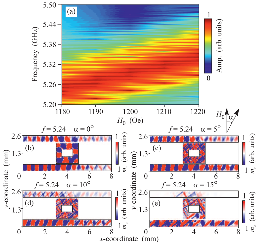
Рис. 4. (Цветной онлайн) (а) – Карта распределения амплитуды ПМСВ в зависимости от частоты и величины внешнего магнитного поля в выходном порте P_2 . (б)–(е) – Карты распределения динамической намагниченности m_z , измеренных на частоте f_1 = 5.24 ГГц при изменении угла внешнего магнитного поля H_0
