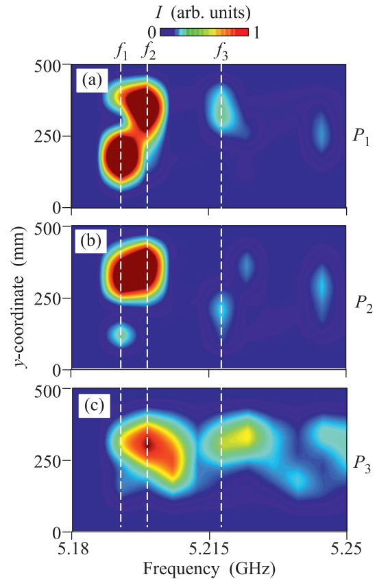
Рис. 3. (Цветной онлайн) Карты распределения интенсивности спиновых волн в области выходных портов P_1 (a), P_2 (b) и P_3 (c)
