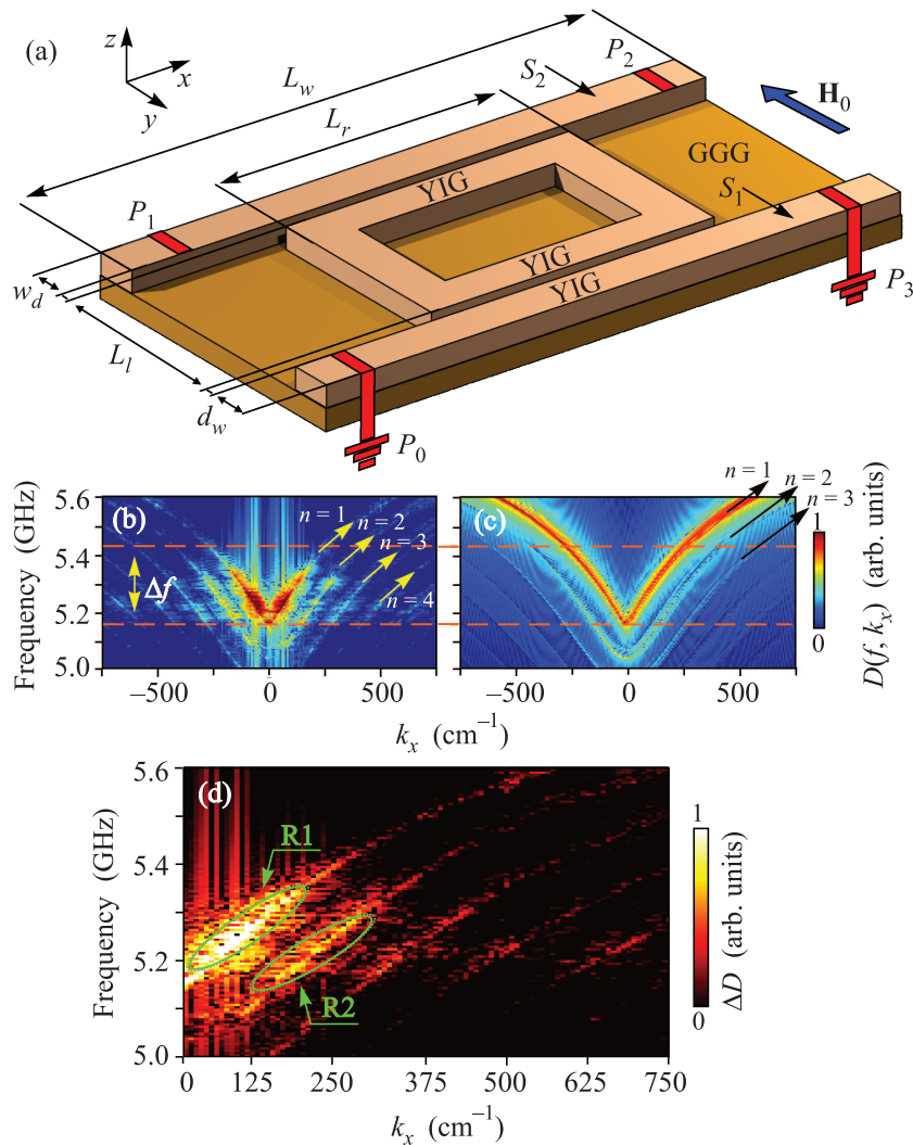
Рис. 1. (Цветной онлайн) (a) – Схематичное изображение исследуемой структуры. (b), (c) – Дисперсионные характеристики ПМСВ распространяющихся в волноводе S_2 (b), S_1 (c), соответственно. (d) – Распределение величины \Delta D на плоскости параметров частота–продольное волновое число
