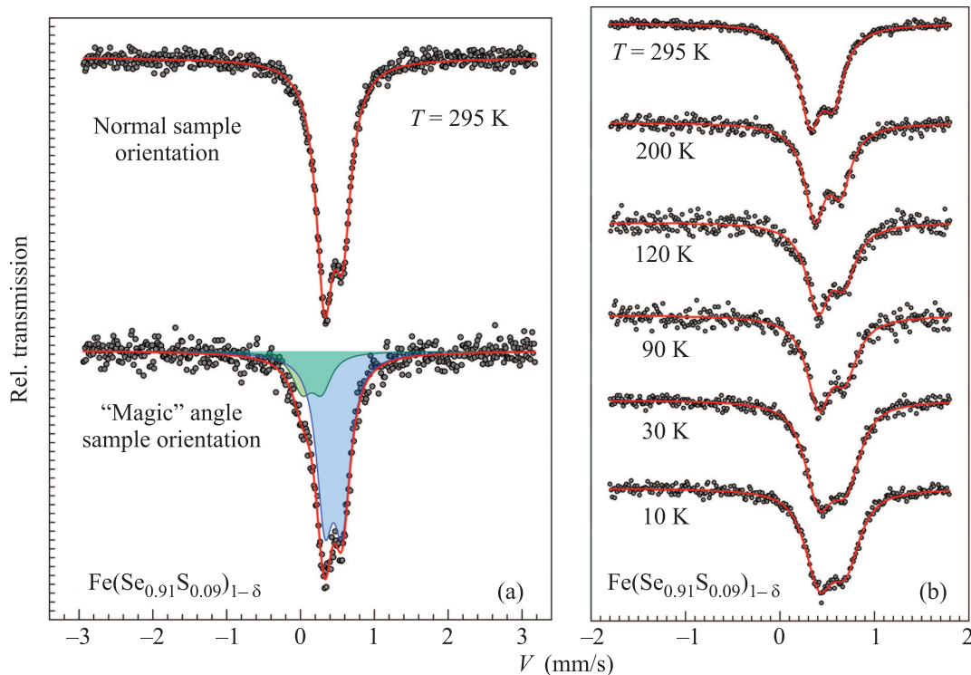
Рис. 3. (Цветной онлайн) Мессбаэровские спектры от монокристалла сверхпроводника \text{Fe}(\text{Se}_{0.91}\text{S}_{0.09})_{1-\delta} : (a) – ориентация образца перпендикулярна к волновому вектору гамма-квантов k_\gamma и для ориентации под “магическим” углом при комнатной температуре; (b) – спектры при различных температурах
