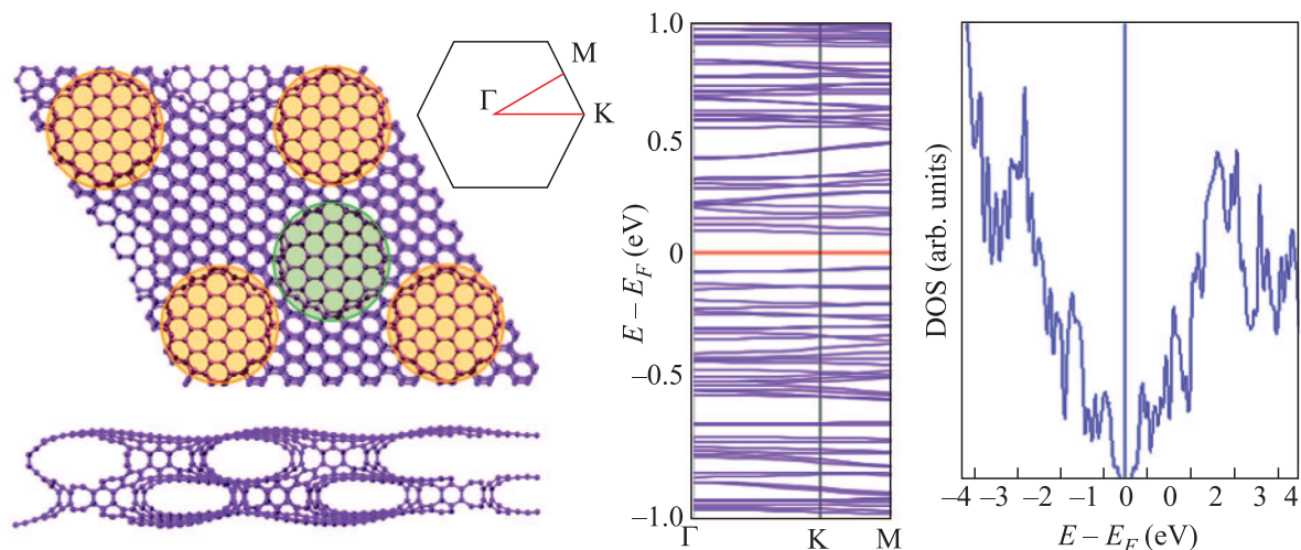
Рис. 3. (Цветной онлайн) Атомная – вид сверху и сбоку по линии разреза – (а), электронная (b) и DOS (c) структуры системы III. Зеленым и желтыми кругами обозначены “замкнутые” нанопоры “1–2” и “2–3” соответственно
