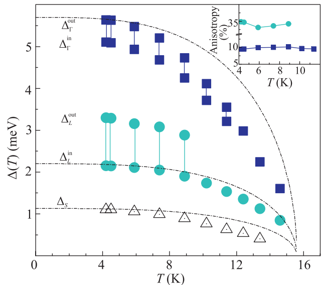
Рис. 4. (Цветной онлайн) Температурные зависимости трех сверхпроводящих щелей в LiFeAs. Индексы in и out определяют пороговые амплитуды для анизотропных щелей. Для сравнения однозонные БКШ-образные кривые показаны штрихпунктиром. На вставке приведены температурные зависимости анизотропии больших щелей \Delta_\Gamma (квадраты) и \Delta_L (кружки), оцененные как 100\% \cdot (1 - \Delta^{\text{in}}/\Delta^{\text{out}})
