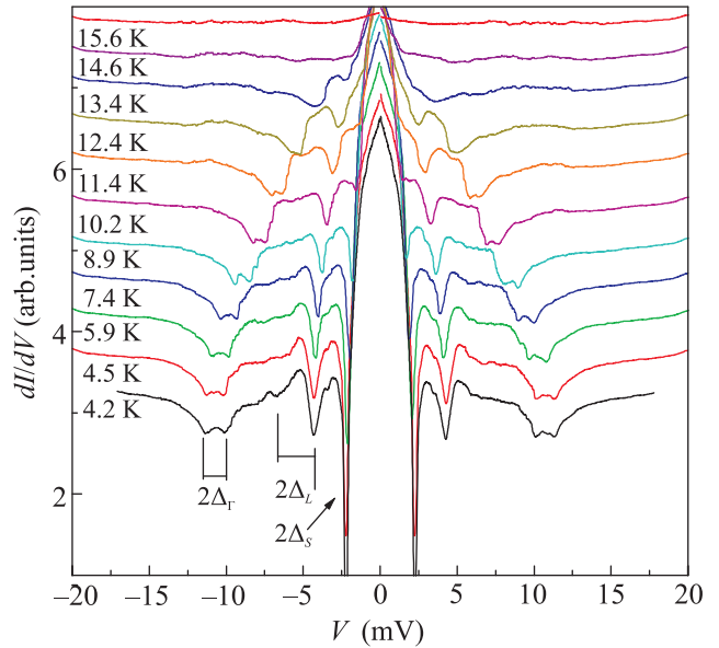
Рис. 2. (Цветной онлайн) Спектры динамической про- водимости андреевского контакта, измеренные при T = 4.2\text{--}15.6 \text{ К} с подавленным нелинейным ходом, со- ответствующим dI(V)/dV -спектру при T_c (показан на вставке a к рис. 1). Кривые сдвинуты вертикально для наглядности. Вертикальные линии и стрелки обозна- чают положения андреевских особенностей, определя- ющие величины трех энергетических параметров \Delta_\Gamma \approx 5.0\text{--}5.7 \text{ мэВ} , \Delta_L \approx 2.1\text{--}3.4 \text{ мэВ} , \Delta_S \approx 1.2 \text{ мэВ} (диа- пазоны значений определяются положениями дублетов на спектрах и соответствуют анизотропии щели)
