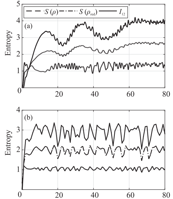
Рис. 2. Временная зависимость энтропии фон Неймана, полученная для двухчастичного состояния двух полей и для каждого поля в отдельности, а также эволюция взаимной информации для двух изначально когерентных полей (а) и двух состояний сжатого вакуума (б) со средним числом \langle N \rangle = 3 и начального состояния атома (13) с \Delta = 0
