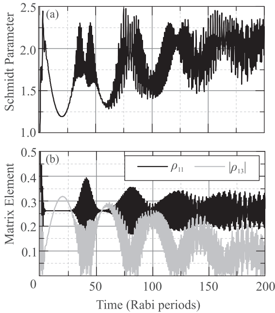
Рис. 1. Временная динамика параметра Шмидта K (a), а также населенности нижнего атомного уровня и недиагонального элемента матрицы плотности атома \rho_{13} (b), полученные при взаимодействии атома в начальном состоянии \phi_{at}(t=0) = \frac{\varphi_1 + \varphi_2}{\sqrt{2}} с когерентными полями с \langle N \rangle = 10
