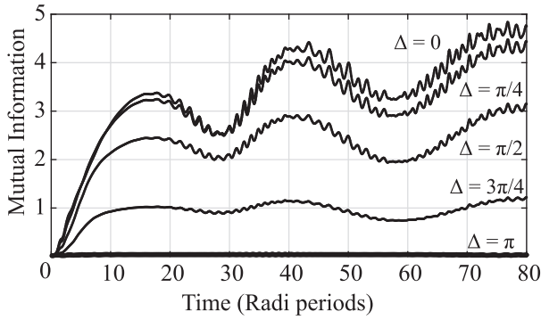
Рис. 3. Временные зависимости взаимной информации двух когерентных полей при различных значениях относительной фазы \Delta между атомными состояниями в начальном условии (13)
