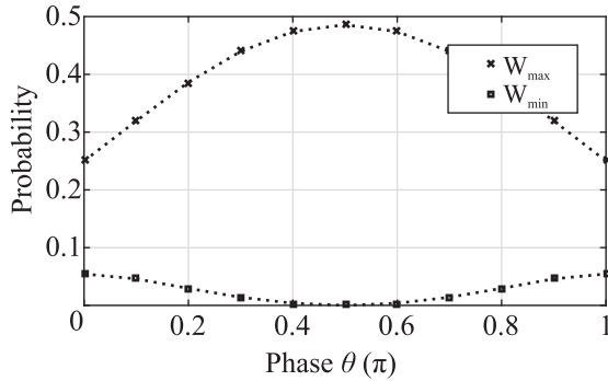
Рис. 5. Зависимость максимального и минимального по времени значений вероятности найти атом в основном состоянии и m фотонов во втором поле в зависимости от фазы пробного поля \theta
