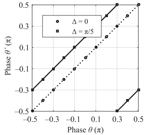
Рис. 4. Относительная фаза \theta' , переданная первому полю, в зависимости от исходной фазы \theta между состояниями второй моды при двух значениях \Delta = 0 и \Delta = \pi/5 в начальном условии для системы (18)
