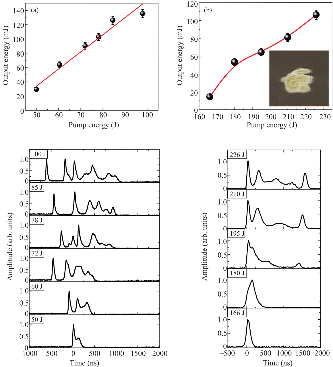
Рис. 4. (Цветной онлайн) Энергия и форма импульса в лазерах Sr:Er:YSGG (a) и Er:YAG (b) с вращающимся зеркалом при различной энергии накачки. На вставке изображен прожиг фотобумаги от пучка в многоимпульсном режиме
