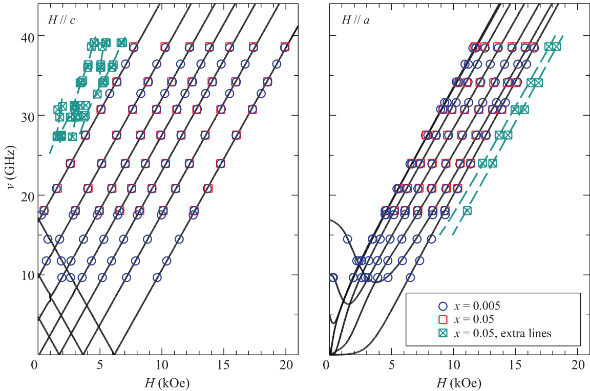
Рис. 3. (Цветной онлайн) Частотно-полевые диаграммы образцов \text{LiY}_{1-x}\text{Gd}_x\text{F}_4 с x = 0.005 (основные линии показаны символами \circ ) и 0.05 ( \square ), полученные при T = 4.2 К для двух основных ориентаций образца во внешнем поле. Символы \boxtimes на обеих панелях соответствуют “дополнительным линиям”, присутствующим только в образце с x = 0.05 . Положения пиков резонансного поглощения, рассчитанные на основе гамильтониана (1) с параметрами, указанными в тексте, показаны сплошными линиями; штриховые линии соответствуют спектрам пар ближайших соседей
