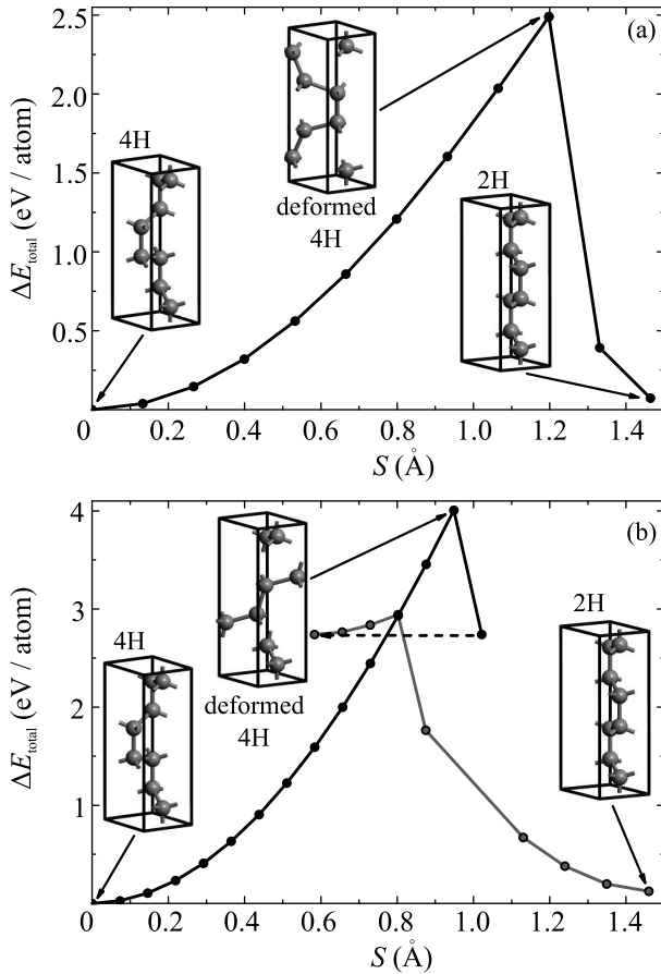
Рис. 1. Графики зависимости разностной полной энергии ( \Delta E_{\text{total}} ) от величины сдвига ( S ) двухатомного молекулярного слоя (а) и при поатомном переносе этого слоя (б) для процесса преобразования 4Н алмаза в 2Н алмаз (значение энергии рассчитано как отношение \Delta E_{\text{total}} для элементарной ячейки к числу перемещаемых атомов)
