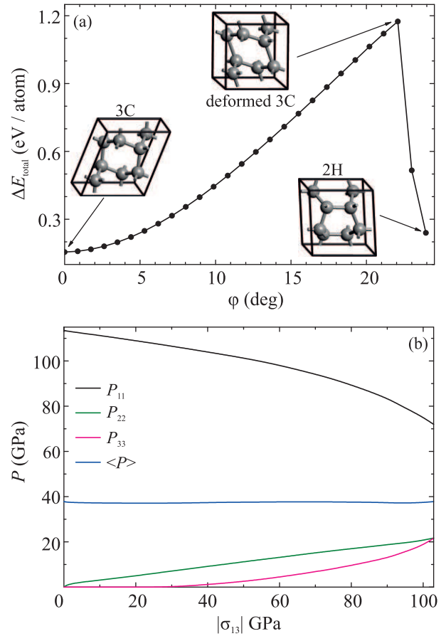
Рис. 2. (Цветной онлайн) (а) – Зависимость разностной полной энергии ( \Delta E_{\text{total}} ) от угла сдвига ( \varphi ) для фазового перехода “3С алмаз \rightarrow 2Н алмаз” (разностные энергии рассчитаны относительно энергии недеформированного 3С алмаза). (б) – Зависимость величин компонент давления от значения модуля сдвигового напряжения \sigma_{13}
