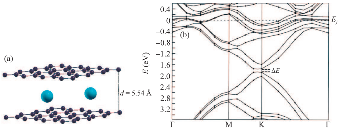
Рис. 5. (Цветной онлайн) (а) – Структура KC_{32} . (б) – Энергетический спектр, соответствующий данной конфигурации. Величина запрещенной зоны составляет \Delta E = 0.1 эВ
