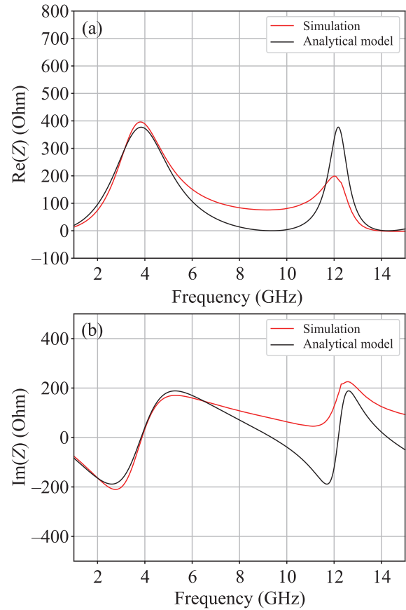
Рис. 2. (Цветной онлайн) Действительная (a) и мнимая (b) часть импеданса, необходимая для идеального согласования, полученная с помощью аналитического расчета и численной модели
