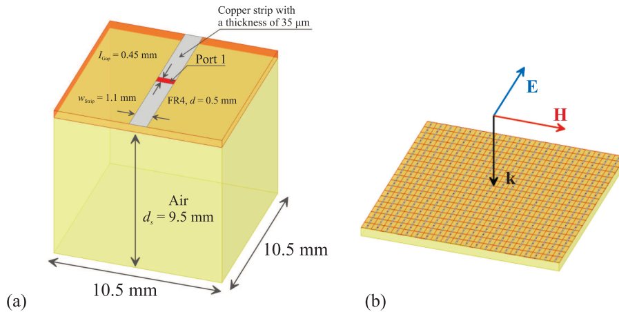
Рис. 1. (Цветной онлайн) (а) – Элементарная ячейка метаматериала (метаатом); (б) – модель образца метаматериала (20 × 20 элементов)
