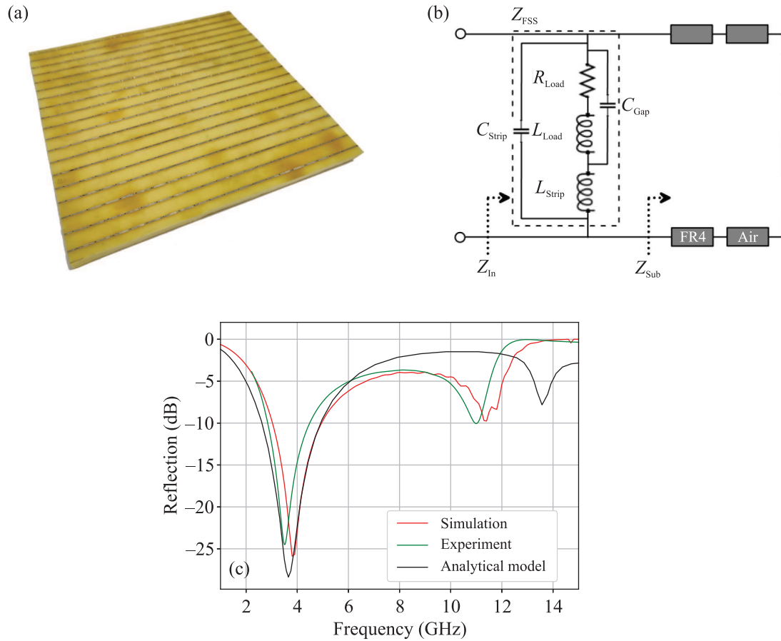
Рис. 3. (Цветной онлайн) (а) – Фотография экспериментального образца метаматериала 20 \times 20 элементов; (б) – эквивалентная схема метаматериала; (с) – коэффициент отражения ЭМ-волны от пассивного поглотителя, полученный с помощью электродинамического моделирования, аналитически и экспериментально
