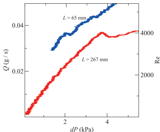
Рис. 1. (Цветной онлайн) Зависимость расхода газа от перепада давления
