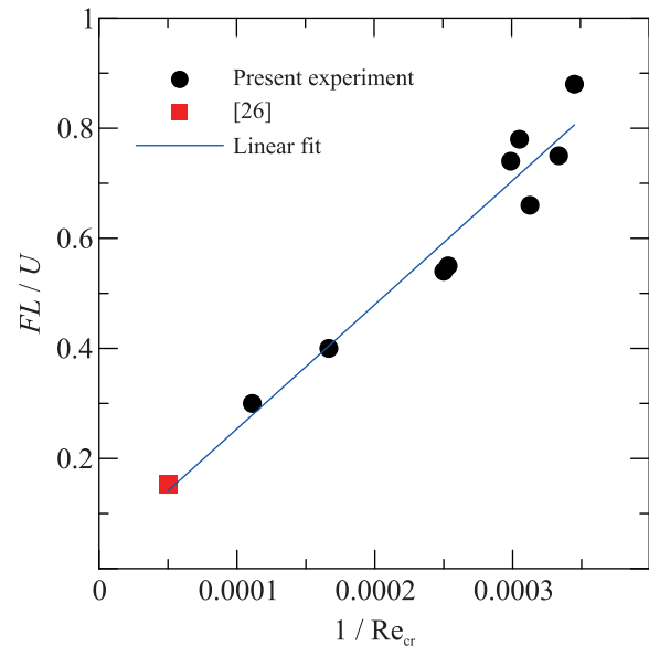
Рис. 4. (Цветной онлайн) Зависимость модифицированного числа Струхала от числа Рейнольдса
