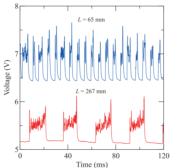
Рис. 2. (Цветной онлайн) Сигнал термоанемометра на выходе из трубы
