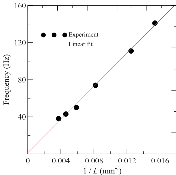
Рис. 3. (Цветной онлайн) Зависимость частоты генерации турбулентных пробок от длины трубы
