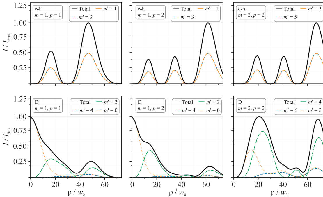
Рис. 2. (Цветной онлайн) Усредненные по углу радиальные профили дифракционной картины второй гармоники. Показана нормированная радиальная зависимость \bar{I}(\rho)/I_{\max} , где \bar{I}(\rho) = \frac{1}{2\pi} \int_0^{2\pi} I(\rho, \varphi) d\varphi – угловое среднее интенсивности излучения на второй гармонике в плоскости детектора на большом расстоянии z ; \rho = \sqrt{x^2 + y^2} . Верхний ряд соответствует сверхпроводнику с электрон-дырочной асимметрией, нижний ряд – сверхпроводнику с диодным эффектом. Три столбца соответствуют падающей ЛГ-накачке с (m, p) = (1, 1) , (1, 2) и (2, 2) ; во всех случаях взята линейная поляризация u_s = u_p = 1/\sqrt{2} . Черная сплошная кривая рассчитана по полному когерентному полю второй гармоники, а цветные кривые показывают вклады отдельных азимутальных каналов m' после углового усреднения: m' = 2m \pm 1 для электрон-дырочного механизма и m' = 2m - 2, 2m, 2m + 2 для диодного механизма
