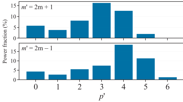
Рис. 3. (Цветной онлайн) Разложение излученного поля второй гармоники по ЛГ-модам для входной моды накачки с индексами (p, m) = (2, 1) в геометрии тонкой сверхпроводящей пленки. Гистограммы показывают долю мощности отдельных выходных ЛГ-каналов на частоте 2\omega в зависимости от радиального индекса p' . Верхняя и нижняя панели соответствуют двум разрешенным по спиральности ветвям орбитального момента: m' = 2m + 1 = 3 и m' = 2m - 1 = 1 . Выбор базиса с характерной шириной w_{2\omega} = w_0/\sqrt{2} соответствует квадратичной природе источника второй гармоники и приводит к конечному набору радиальных мод p' = 0, 1, \dots, 2p + 2 . Таким образом, рисунок демонстрирует не только правило отбора по азимутальному индексу m' = 2m \pm 1 , но и конечную структуру возбужденных радиальных ЛГ-мод.
