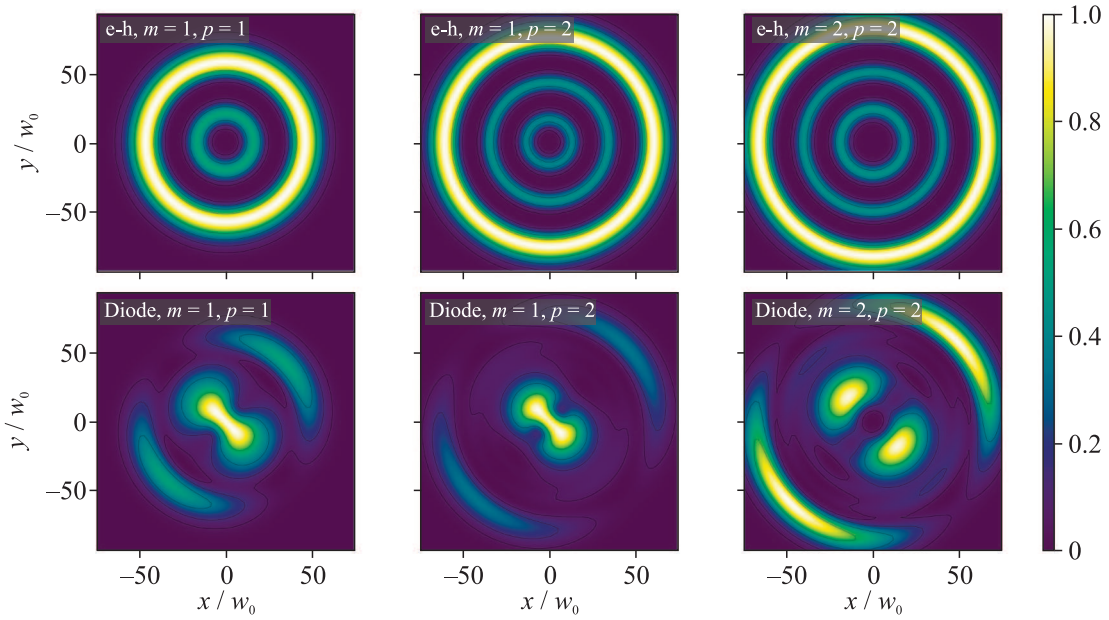
Рис. 1. (Цветной онлайн) Дифракционные картины излучения на второй гармонике, создаваемого фотоиндуцированными токами в тонкой пленке. Показана нормированная интенсивность I(x, y)/I_{\max} в плоскости детектора на большом расстоянии z . Верхний ряд соответствует сверхпроводнику с электрон-дырочной асимметрией, нижний ряд – сверхпроводнику с диодным эффектом. Столбцы соответствуют (m, p) = (1, 1), (1, 2), (2, 2) . Во всех панелях взята ЛГ-накачка с линейной поляризацией u_s = u_p = 1/\sqrt{2} . В диодном случае для m = 1 присутствует канал m' = 0 , что допускает ненулевую интенсивность в центре картины, тогда как для m = 2 разрешены только m' = 2, 4, 6 , и интенсивность в центре картины подавлена.
