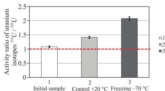
Рис. 1. (Цветной онлайн) Изотопное отношение ^{234}\text{U}/^{238}\text{U} в различных фазах эксперимента. 1 – Исходная проба: исходное отношение в твердой фазе. 2 – Контроль +20^\circ\text{C} : жидкая фаза после изотермического выщелачивания; 3 – Замораживание -70^\circ\text{C} : жидкая фаза после трех циклов замораживания-оттаивания. Красная пунктирная линия обозначает уровень векового радиоактивного равновесия ^{234}\text{U}/^{238}\text{U} = 1.00
