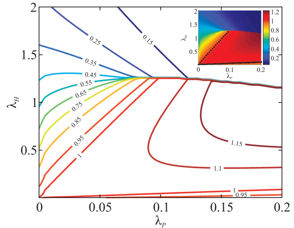
Рис. 1. (Цветной онлайн) Эффективное обменное взаимодействие J_{gg'}^{00} коррелированных поляронов с сильной электрон-фононной связью в единицах J_{gg'}^{00} ( \lambda_H = \lambda_P = 0 ). Взаимодействие носителей заряда с решеткой характеризуется двумя типами электрон-решеточной связи: Хольштейна \lambda_H и Пайерлса (Су–Шриффера–Хигера) \lambda_P . На вставке величина обмена показана цветом, цветовая шкала соответствует основному рисунку, непременормированный контур выделен черным пунктиром
