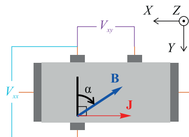
Рис. 1. (Цветной онлайн) Схематическое представление образца и геометрии измерения ПЭХ и АМС в плоскости XY четырехзондовым методом
