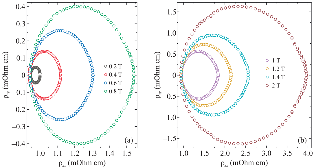
Рис. 3. (Цветной онлайн) Семейство параметрических кривых, демонстрирующих зависимость \rho_{xy} от \rho_{xx} при T = 80 К в разных магнитных полях
