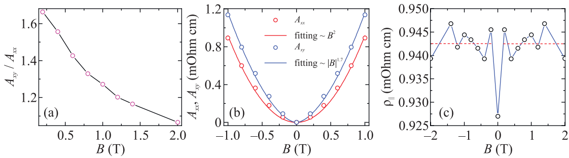
Рис. 4. (Цветной онлайн) (а) – Зависимость отношения амплитуд ПЭХ и АМС \frac{A_{xy}}{A_{xx}} от магнитного поля. (b) – Магнитополевая зависимость амплитуд A_{xx} и A_{xy} в слабых полях (0.2–1) Тл, удовлетворяющих критерию 0.75 B < 1 . Символы – эксперимент, сплошные кривые – подгонка квадратичным ( A_{xx} \sim B^2 ) и степенным ( A_{xy} \sim |B|^{1.7} ) законом. (с) – Магнитосопротивление \rho_{||} при разных значениях параллельного магнитного поля (символы). Пунктирная линия – среднее значение \rho_{||} в интервале (0.2–2) Тл. Также приведено удельное сопротивление в нулевом поле \rho_0 = 9.27 \times 10^{-4} Ом см
