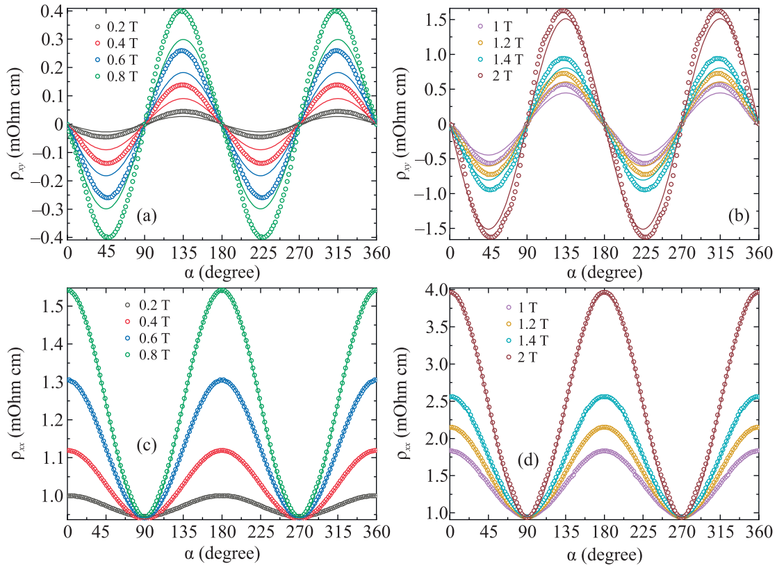
Рис. 2. (Цветной онлайн) Планарный магнитотранспорт в ультрочином образце HgSe при T = 80 K в слабых магнитных полях. (а), (б) – Угловая зависимость удельного планарного холловского сопротивления \rho_{xy}(\alpha) в разных магнитных полях. Символы – эксперимент, сплошные линии – подгонка по формуле (1) с использованием амплитуды для АМС. (с), (д) – Угловая зависимость удельного планарного АМС \rho_{xx}(\alpha) в разных магнитных полях. Символы – эксперимент, сплошные линии – подгонка по формуле (2)
