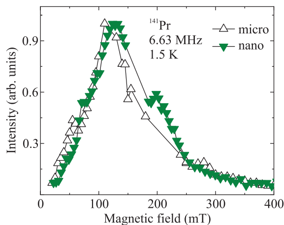
Рис. 1. (Цветной онлайн) Спектр ядер ^{141}\text{Pr} в микро- и наноразмерном порошках \text{PrF}_3 на частоте 6.63 МГц в магнитных полях 0–400 мТл при температуре 1.5 K
