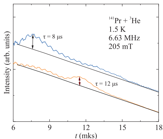
Рис. 3. (Цветной онлайн) Сигнал спинового эха ядер ^{141}\text{Pr} в контакте с жидким гелием-3
