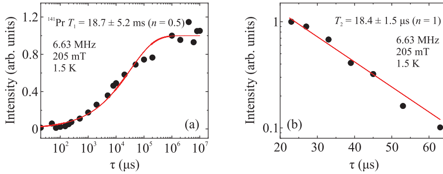
Рис. 4. (Цветной онлайн) Кривые восстановления продольной (а) и спада поперечной (б) намагниченности ядер ^{141}\text{Pr} в наноразмерном порошке \text{PrF}_3 на частоте 6.63 МГц в магнитном поле 205 мТл в контакте с жидким гелием-3
