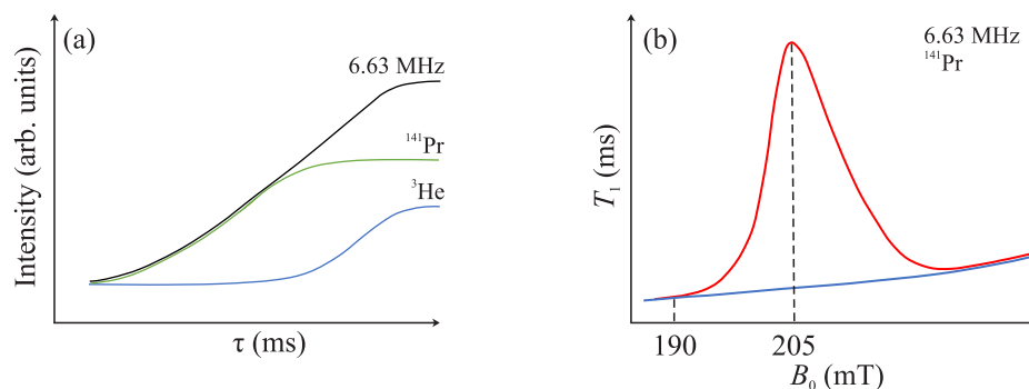
Рис. 2. (Цветной онлайн) Разделение вкладов ядер ^{141}\text{Pr} и ^3\text{He} в восстановление продольной намагниченности, использованное в статье [23] (a) и резонансное изменение времен T_1 релаксации ^{141}\text{Pr} в магнитных полях 190–220 мТл (b)
