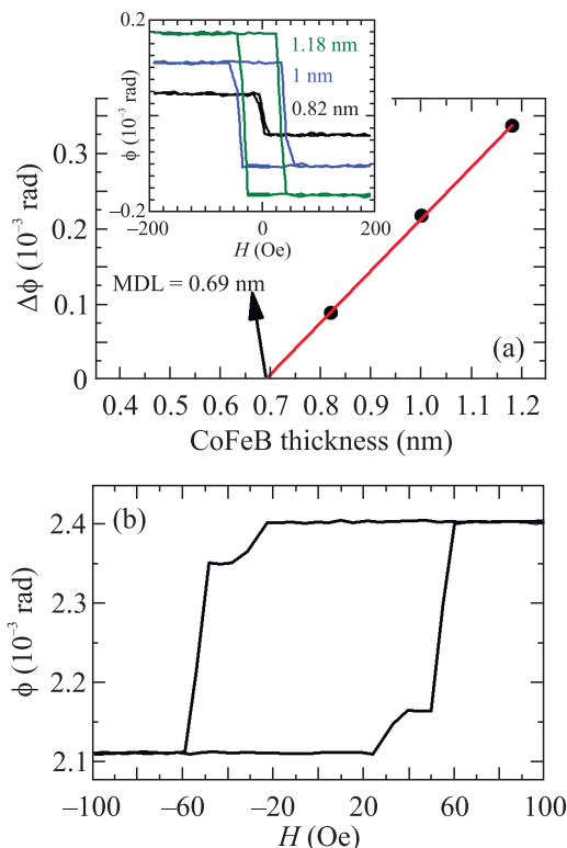
Рис. 1. (Цветной онлайн) (а) – Зависимость полярного эффекта Керра от толщины магнитной пленки в структуре W(3)/CoFeB( t )/MgO(2). На вставке – петли гистерезиса для структур с разной толщиной магнитного слоя. (б) – Гистерезис перемагничивания двухслойной структуры W(3)/CoFeB(1.1)/MgO(2)/CoFeB(1.5)/W(3) (после отжига)
