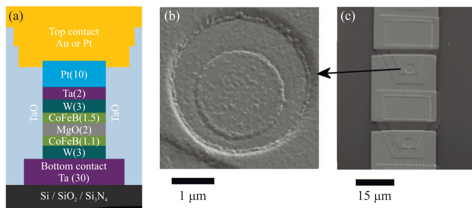
Рис. 2. (Цветной онлайн) (a) – Структура слоев ТМК. (b) – Изображение круглого ТМК контакта и (c) изображение участка цепочки ТМК в растровом электронном микроскопе
