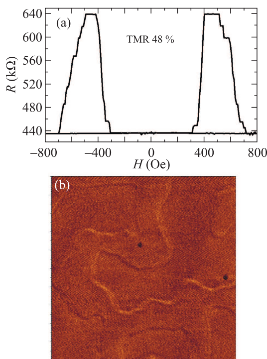
Рис. 3. Цветной онлайн) (a) – Полная кривая магнитосопротивления цепочки ТМК после отжига при приложенном напряжении 10 мВ. (b) – МСМ-изображение магнитных доменов в исходной многослойной ТМР структуре. Размер скана 10 × 10 мкм 2
