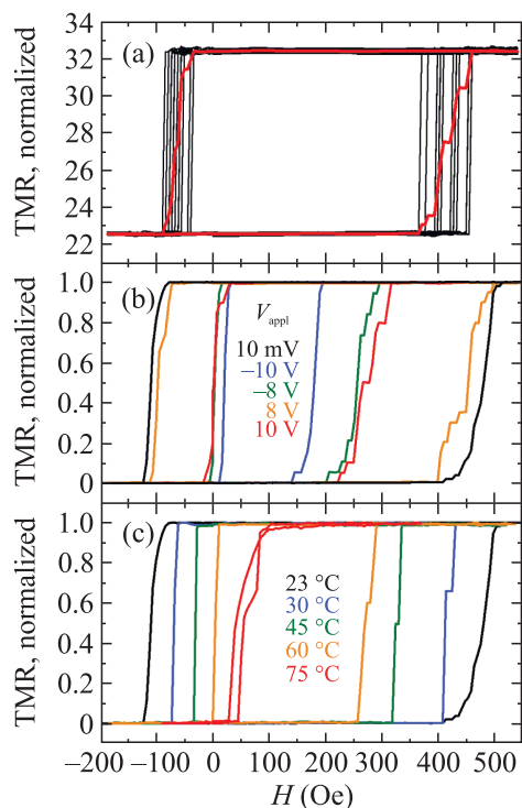
Рис. 4. (Цветной онлайн) (а) – Петли перемагничивания низкокоэрцитивного слоя туннельного контакта при напряжении 10 мВ. Толстой пунктирной линией показана усредненная по 30 проходам петля перемагничивания. (б) – Усредненные петли перемагничивания низкокоэрцитивного слоя туннельного контакта при подаче импульсов напряжения разной величины и полярности. (с) – Петля перемагничивания низкокоэрцитивного слоя туннельного контакта при разных температурах при напряжении 10 мВ
