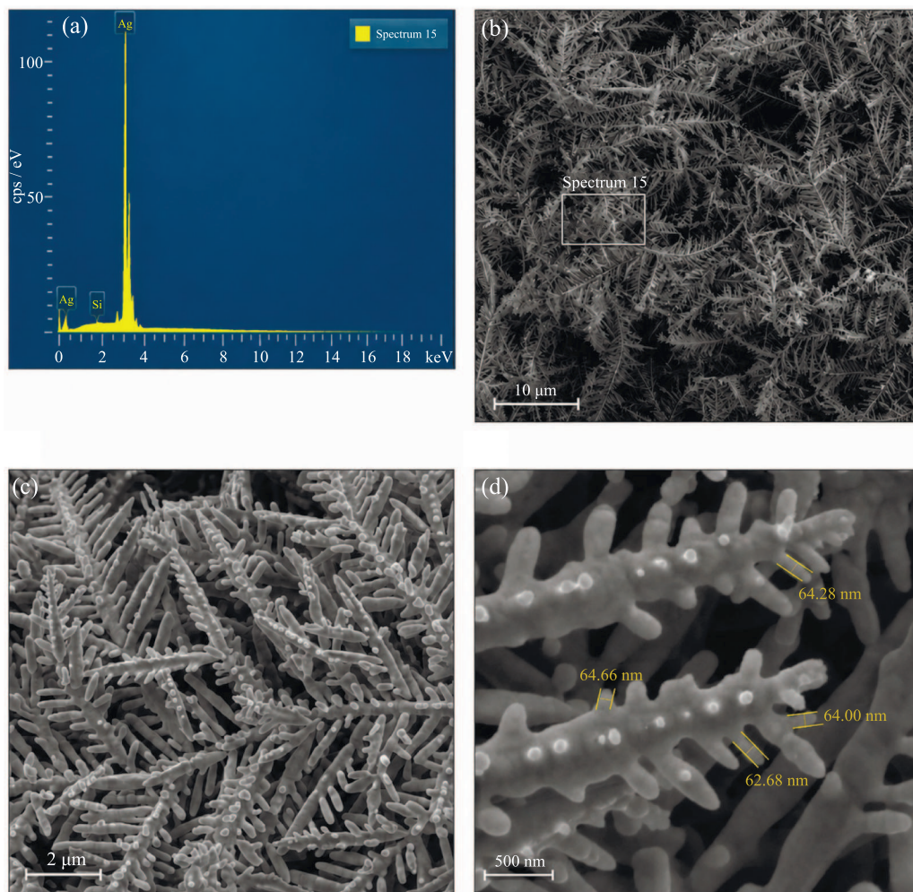
Рис. 1. (Цветной онлайн) Рентгеновский спектр ЭДС и СЭМ изображения комплексов “Ag-дендриты”, сформированных в растворе 4.8 М HF и 0.005 М AgNO 3 на 5 мл H 2 O
