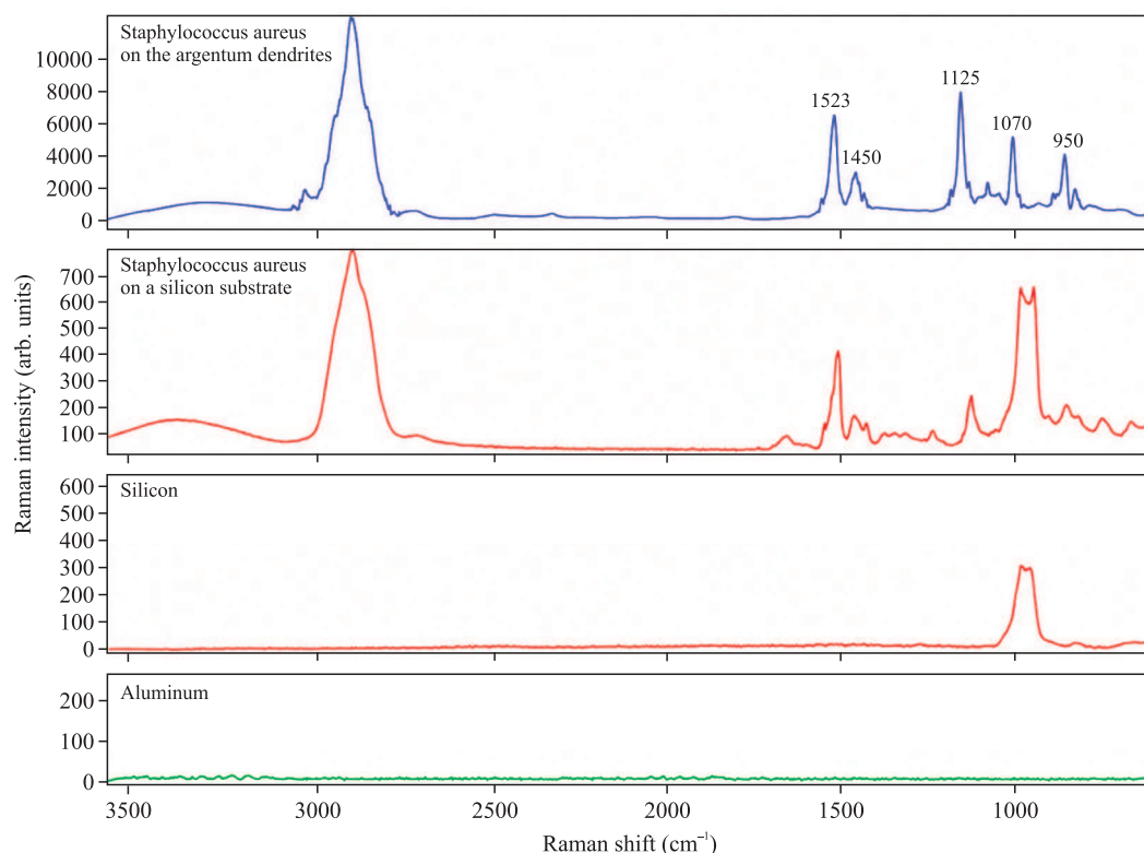
Рис. 2. (Цветной онлайн) Спектры комбинационного рассеяния (сверху вниз) бактерии Staphylococcus aureus на серебряных дендритах и на кремниевой подложке, а также спектры кремния и алюминия в отдельности
