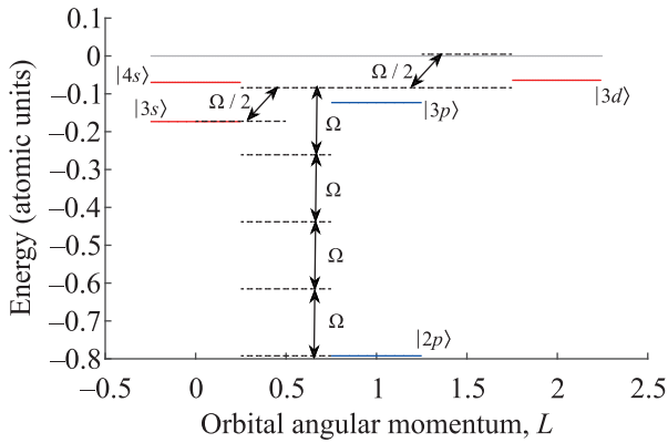
Рис. 2. (Цветной онлайн) Энергетическая диаграмма низших связанных состояний атома Ne в модели (7). Красными горизонтальными линиями обозначены положения энергий четных состояний, синими линиями – нечетных состояний, серой линией – невозмущенный потенциал ионизации атома. Длинная двойная стрелка обозначает энергию фотона УФ поля частоты \Omega , короткая двойная стрелка – энергию фотона субгармоники частоты \Omega/2
