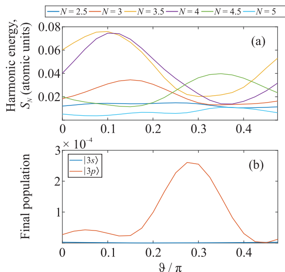
Рис. 7. (Цветной онлайн) Зависимости: (a) – энергий компонент в спектре второй производной индуцированного дипольного момента атома Ne на частотах N\Omega , S_N , и (b) – финальной населенностей низших возбужденных состояний от фазовой задержки поля субгармоники \vartheta , полученные в рамках модели (7). Интенсивность УФ поля I_\Omega = 1.6 \times 10^{14} Вт/см 2 , интенсивность поля субгармоники I_{\Omega/2} = 5.66 \times 10^{13} Вт/см 2
