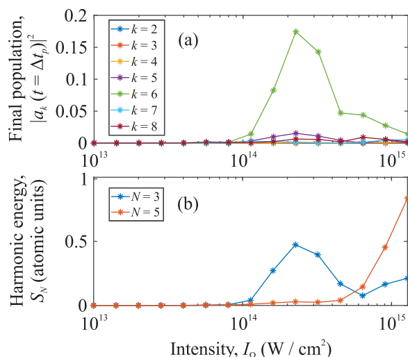
Рис. 3. (Цветной онлайн) Зависимости (а) финальной (по окончании лазерного импульса) населенности низших возбужденных состояний атома Ne, |a_k|^2 , k = 2, \dots, 8 (см. рис. 1), а также (б) энергий 3-й и 5-й гармоник, S_N , от интенсивности УФ импульса частоты \Omega = 0.1769 ат. ед. ( \lambda_{UV} = 257.5 \text{ nm} ), полученные в рамках модели (3)
