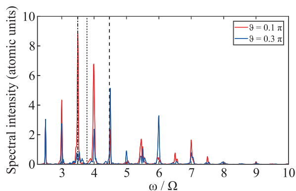
Рис. 8. (Цветной онлайн) Спектры второй производной индуцированного дипольного момента атома Ne (6b) в двухчастотном поле (1), рассчитанные в рамках модели (7). I_\Omega = 1.6 \times 10^{14} Вт/см 2 , I_{\Omega/2} = 5.66 \times 10^{13} Вт/см 2 . Красная и синяя кривые соответствуют значениям \vartheta = 0.1\pi и \vartheta = 0.3\pi . Вертикальными штриховой, пунктирной и штрихпунктирной линиями обозначены положения невозмущенного потенциала ионизации и невозмущенных энергий возбуждения состояний |3p\rangle и |3s\rangle соответственно
