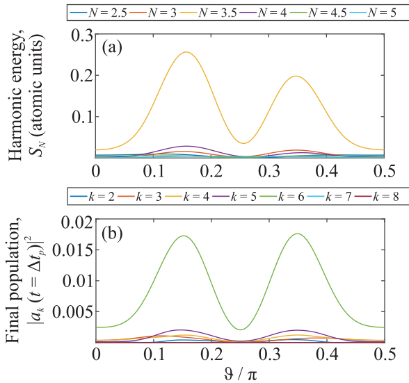
Рис. 6. (Цветной онлайн) Зависимости: (а) – энергий компонент в спектре второй производной индуцированного дипольного момента атома Ne на частотах N\Omega , S_N , и (б) – финальных (после окончания импульса) населенностей низших возбужденных состояний, |a_k|^2 , k = 2, \dots, 8 (см. рис. 1), от фазовой задержки поля субгармоники \vartheta , полученные в рамках модели (3). Интенсивность УФ поля I_\Omega = 1.6 \times 10^{14} Вт/см 2 , интенсивность поля субгармоники I_{\Omega/2} = 4 \times 10^{13} Вт/см 2
