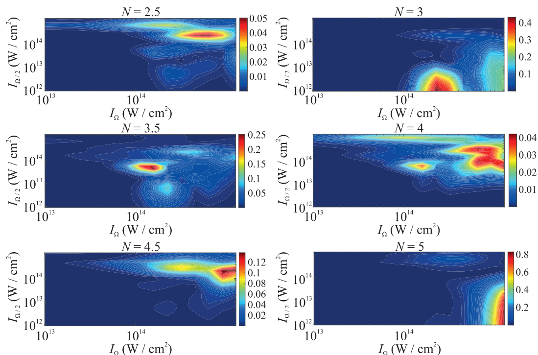
Рис. 5. (Цветной онлайн) Зависимости энергии низших гармоник в спектре второй производной дипольного момента атома Ne от интенсивностей спектральных компонент лазерного поля (1), I_\Omega ( \lambda_{UV} = 257.5 нм) и I_{\Omega/2} ( \lambda_{VIS} = 515 нм), при значении \vartheta = 0.15\pi , полученные в рамках модели (3)
