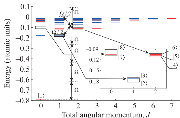
Рис. 1. (Цветной онлайн) Энергетическая диаграмма связанных состояний атома Ne, которые учитывались в модели (3). Красными горизонтальными линиями обозначены положения энергий четных состояний, синими линиями – нечетных состояний, серой линией – невозмущенный потенциал ионизации атома. Двойная стрелка большей длины обозначает энергию фотона УФ поля частоты \Omega , короткая двойная стрелка – энергию фотона субгармоники видимого диапазона частоты \Omega/2 . На вставке изображены энергии низших возбужденных связанных состояний, которые заселяются в линейно поляризованном лазерном поле в результате переходов из основного состояния. Основное и низколежащие возбужденные состояния на вставке обозначены номерами |k\rangle , k = 1, \dots, 8
