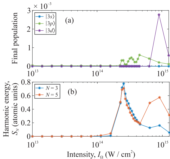
Рис. 4. (Цветной онлайн) Зависимости: (а) – финальной населенности низших возбужденных состояний атома Ne и (б) – энергий 3-й и 5-й гармоник от интенсивности лазерного поля при \Omega = 0.1769 ат. ед. ( \lambda_{UV} = 257.5 нм), полученные в рамках модели (7)
