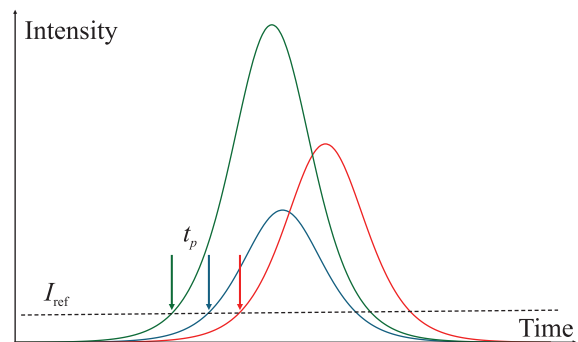
Рис. 4. (Цветной онлайн) Иллюстрация разброса времени задержки импульсов сверхизлучения
