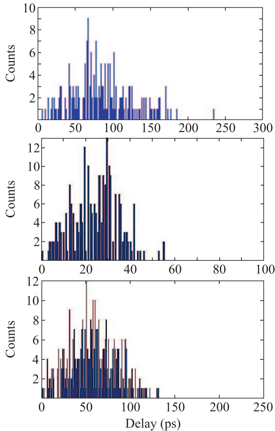
Рис. 3. (Цветной онлайн) Количество отсчетов в зависимости от относительной задержки между максимумами импульсов сверхизлучения и опорного импульса для трех гетероструктур. Значения среднего времени задержки и среднеквадратичного отклонения составляют 71, 28, 63 и 32, 29, 31 пс соответственно
