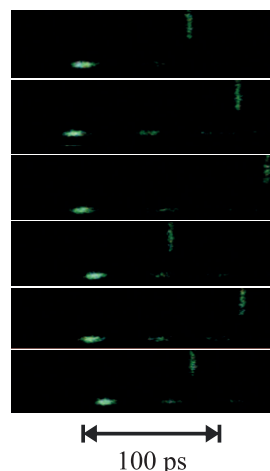
Рис. 2. (Цветной онлайн) Исходные изображения, полученные с экрана стрик-камеры и иллюстрирующие флуктуации относительной задержки между импульсами сверхизлучения (бледная вертикальная полоса вверху) и импульсами опорного лазера (яркая горизонтальная полоса внизу)
