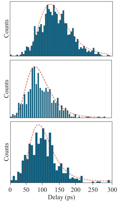
Рис. 5. (Цветной онлайн) Аппроксимация экспериментальных данных функцией (2) для 3 сверхизлучающих гетероструктур. Значения среднего времени задержки и среднеквадратичного отклонения составляют 142, 99, 98 и 43, 35, 38 пс соответственно
