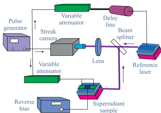
Рис. 1. (Цветной онлайн) Схема эксперимента
