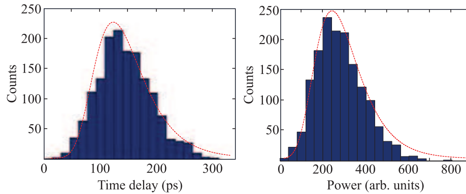
Рис. 6. (Цветной онлайн) Слева – распределение времени задержки фемтосекундных импульсов сверхизлучения, полученные с помощью стробоскопического осциллографа. Значения среднего времени задержки и среднеквадратичного отклонения составляют 147 и 52 пс. Справа – флуктуации их пиковой мощности. Красные пунктирные линии – аппроксимации функцией (2)
