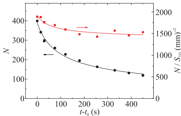
Рис. 3. (Цветной онлайн) Зависимость числа топологических дефектов N (черные кружки, левая ось) и плотности дефектов N/S_{2D} (красные квадраты, правая ось) в двумерной капле из дефектов от времени. S_{2D} – площадь капли. Точность определения количества дефектов порядка размера точек. Число дефектов со временем уменьшается, плотность дефектов практически не изменяется при t - t_0 > 100 с
