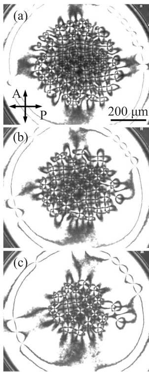
Рис. 2. Трансформация двумерной капли из дефектов. Количество дефектов уменьшается со временем: (а) – N = 297 ; (б) – N = 195 ; (с) – N = 119 . Площадь, занимаемая каплей, также уменьшается. Фотографии (б) и (с) сделаны через 150 и 420 с после фото (а). Двумерная капля из дефектов получена при охлаждении со скоростью 0.3^\circ\text{C}/\text{мин}
