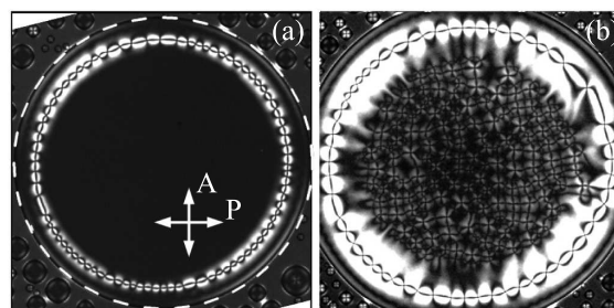
Рис. 1. (a) – Большая изотропная капля в нематическом окружении с круглой цепочкой из +1 и -1 топологических дефектов. Маленькие изотропные капли также видны у краев фотографии. (b) – Двумерная капля из топологических дефектов образуется внутри цепочки при охлаждении. Горизонтальный размер фотографии 815 мкм. Толщина оптической ячейки 40 мкм. Число топологических дефектов в цепочках 84 (a) и 56 (b), в двумерной капле из дефектов внутри цепочки 415 (b). Пунктирная линия на (a) обозначает границу изотропной капли
