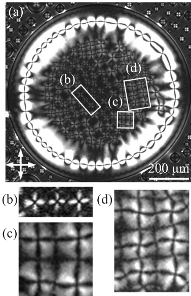
Рис. 4. (a) – Капля из топологических дефектов. Кластеры из упорядоченных дефектов обведены прямоугольниками. Внизу в увеличенном масштабе приведены линейный (b), квадратный (c) и прямоугольный (d) кластеры. Горизонтальные размеры: (b) – 147 мкм; (c) – 80 мкм; (d) – 110 мкм
