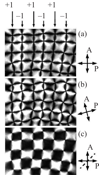
Рис. 5. Фрагмент упорядоченного кластера из топологических дефектов. Фотографии, сделанные со скрещенными поляризаторами (P – поляризатор, A – анализатор), ориентированными параллельно и перпендикулярно горизонтальной оси (a), со скрещенными поляризаторами, повернутыми на 15^\circ против часовой стрелки (b), с оптическим компенсатором (c) позволяют определить знаки топологических дефектов. Стрелки в верхней части рисунка указывают +1 и -1 топологические дефекты в верхнем ряду. Соседние дефекты имеют противоположные знаки. Пунктирная линия в правой части рисунка показывает ориентацию медленной оси компенсатора. Горизонтальный размер фотографий 170 мкм
