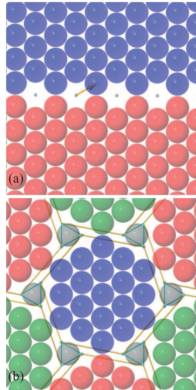
Рис. 1. (Цветной онлайн) (а) – Одиночный сбой упаковки и (б) – пример сети протяженных дефектов в системе жестких дисков [15]
