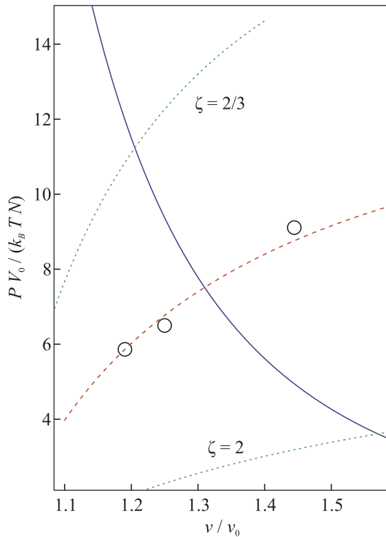
Рис. 3. (Цветной онлайн) Определение точки плавления системы жестких дисков (см. текст). Черные кружки и красная штриховая кривая отвечают двум равенствам формулы (5). Синяя кривая – уравнение состояния системы жестких дисков, в качестве которого взято вириальное разложение по степеням плотности. Зеленые пунктирные кривые отвечают формуле (6) с двумя различными параметрами \zeta
