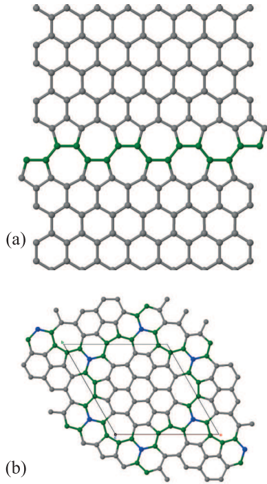
Рис. 2. (Цветной онлайн) (а) – Одиночный сбой упаковки и (b) – пример сети протяженных дефектов максимальной концентрации в графене [23]
