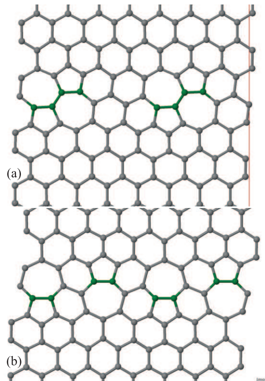
Рис. 5. (Цветной онлайн) Примерная структура “прерывистого” сбоя упаковки, состоящего из изолированных дефектов Стоуна–Вейлса (а) и диссоциированных дефектов Стоуна–Вейлса (b), описываемого формулой (9)
