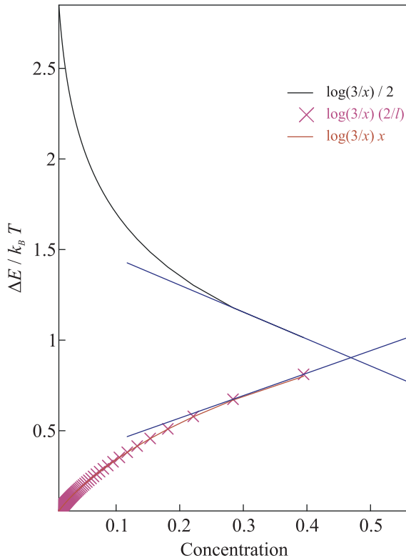
Рис. 4. (Цветной онлайн) Определение точки плавления графена. Символы \times и красная кривая соответствуют двум равенствам формулы (8). Черная кривая – “уравнение состояния” в твердой фазе отвечает формуле (9)
