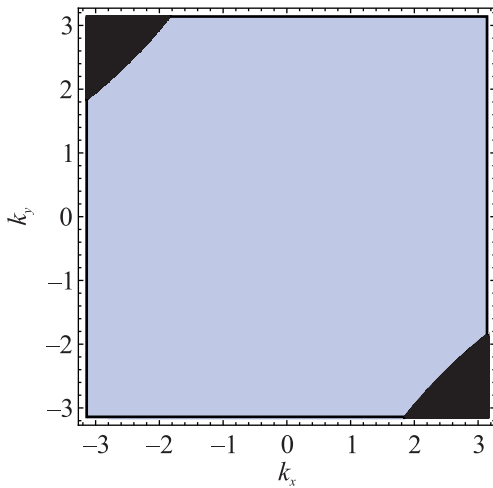
Рис. 2. (Цветной онлайн) Области существования нетопологических и топологических ПСС в нашей модели. Топологически тривиальным ПСС соответствует серая (светлая) область. Топологически нетривиальным ПСС – черная (темная) область. По осям отложены k_x и k_y (зона Бриллюэна), z_c = 3
