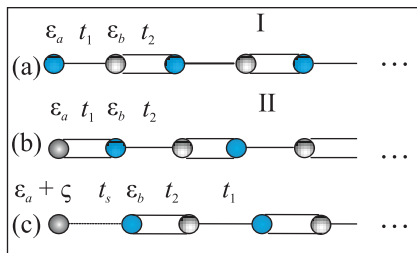
Рис. 1. (Цветной онлайн) Одномерные базовые модели сильной связи, рассматриваемые в настоящей работе. I – топологически нетривиальный 1D кристалл, II – топологически тривиальный 1D кристалл
