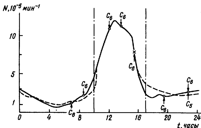
Рис. 2. Изменение скорости счета радиоимпульсов N в течение суток. \circ — совпадения при работе управляющей установки O_I и антенны A_I (сплошная кривая); \times — совпадения при работе управляющей установки O_2 и антенны A_2 (штриховая кривая); C_5, C_6 — совпадения в схеме 5 или 6 соответственно; штрих-пунктирной линией выделен интервал времени возникновения амплитудных перегрузок оконечного усилителя
