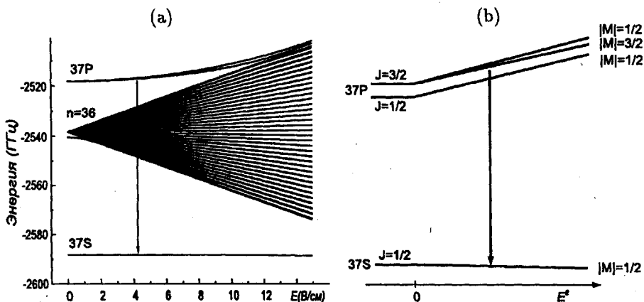
Рис.1. а) Расчетная штарковская диаграмма ридберговских уровней в атомах \text{Na} для состояний с |M| = 1/2 ; б) схема микроволнового перехода 37P - 37S в электрическом поле
